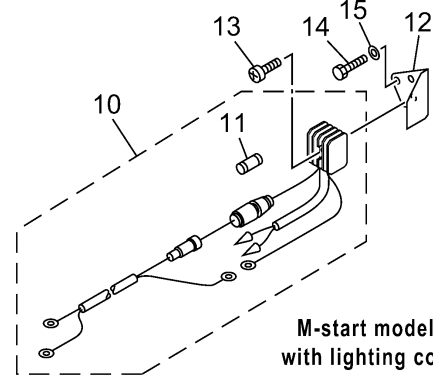
RECTIFIER KIT
